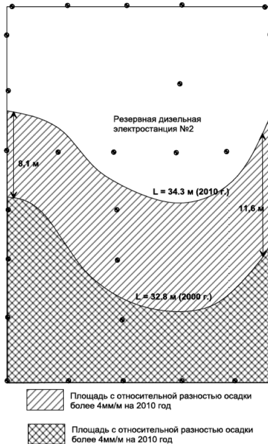
Рисунок Р.8 – Схема определения скорости распространения зоны с относительной разностью < 4 \text{ мм/м}
